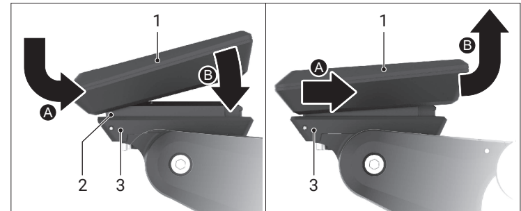
Fig. : 22 Montage de l'ordinateur de commande Kiox 300
