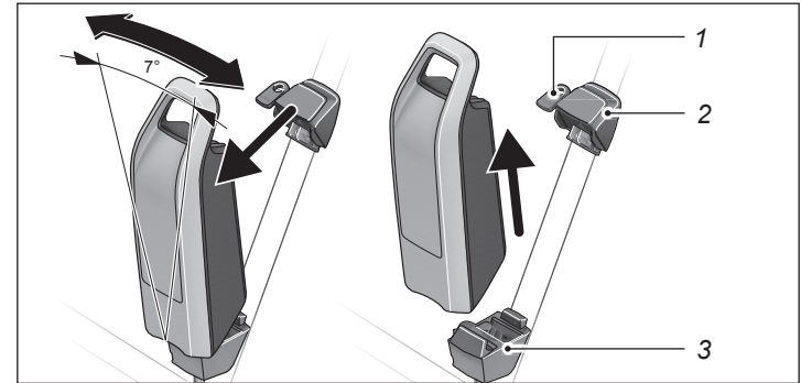
Abb. Rahmenakku (exemplarisch)
