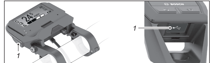
Abb. USB-Anschluss am „SmartphoneHub“ und am „Kiox“
