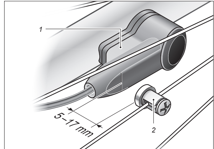
Abb. Geschwindigkeitssensor
