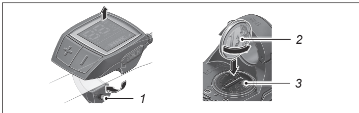
Abb. Batteriewechsel
