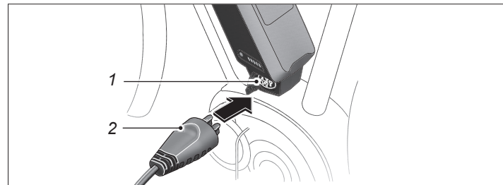
Abb. Eingesetzter Akku (exemplarisch)
