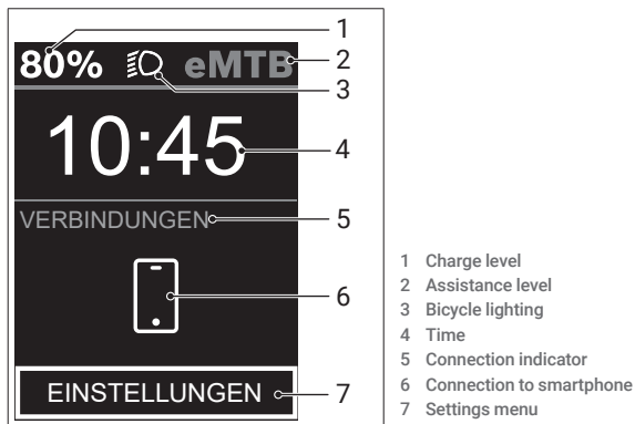
Fig.: 26 Kiox 300 status screen
